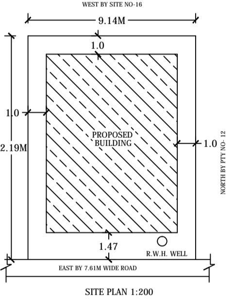
SITE PLAN 1:200
